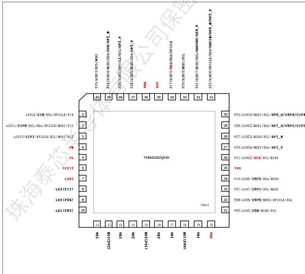
图 1 - TX8M2262QF40 (QFN40) 封装图
