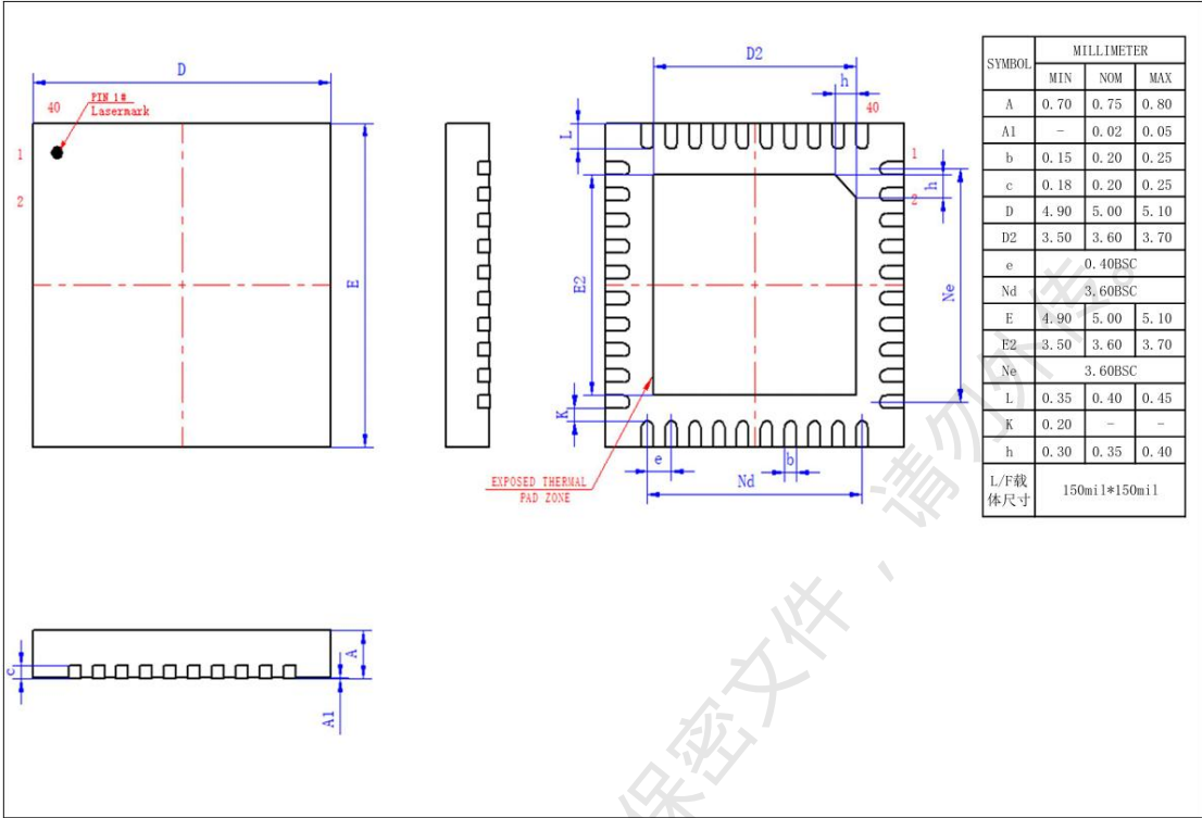
图 3- QFN40 封装 POD 图
